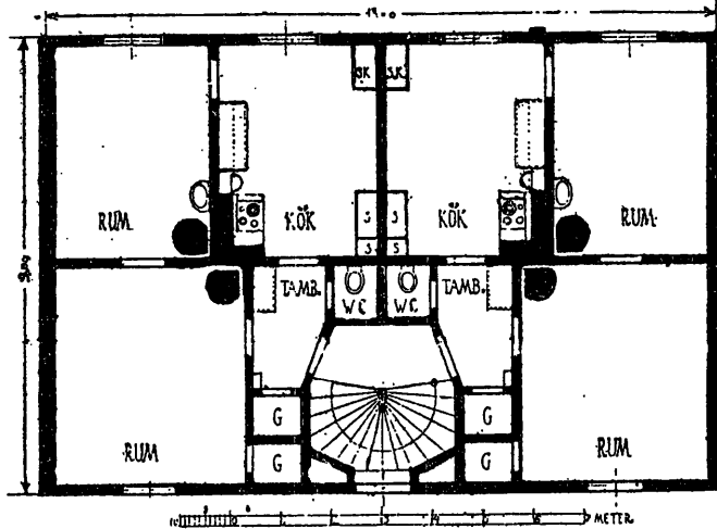
Planritning till en mindre 2-rumslägenhet.
